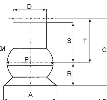
позиция / Pos. 4
