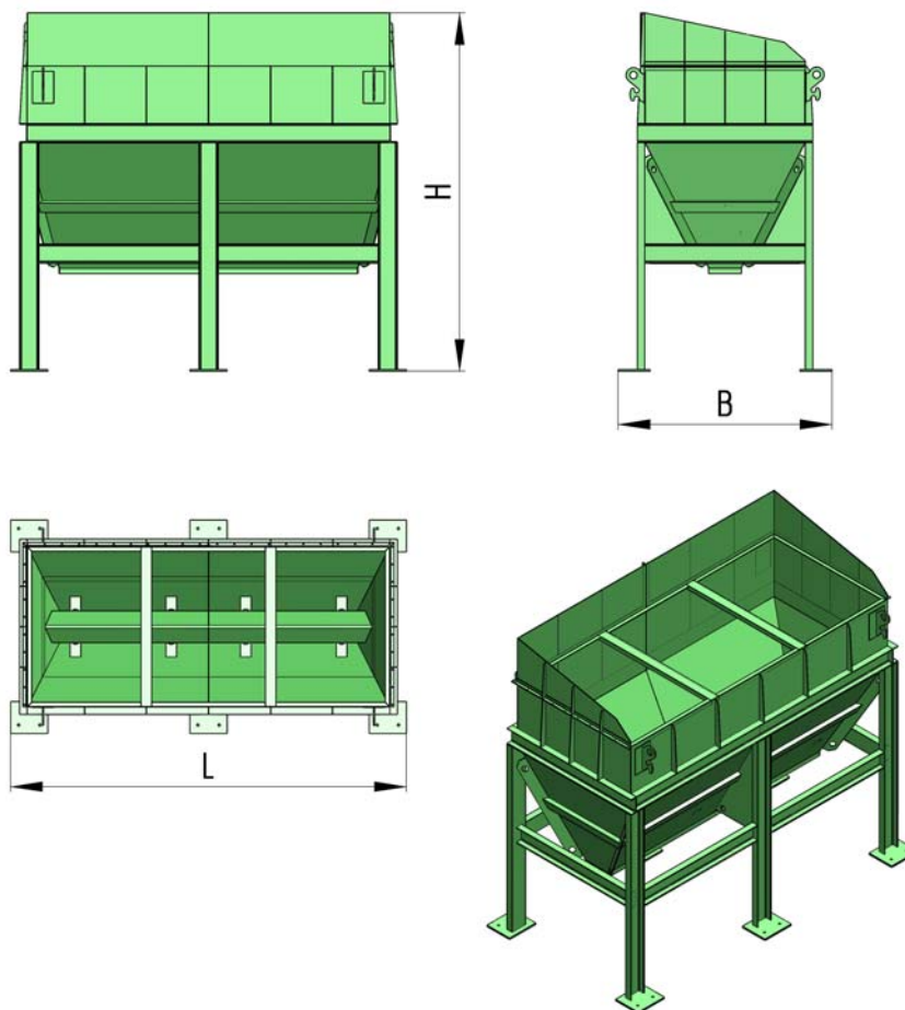
Бункер для песка с вибратором и нижним транспортером выдачи на заводе газобетона (рабочее состояние)
